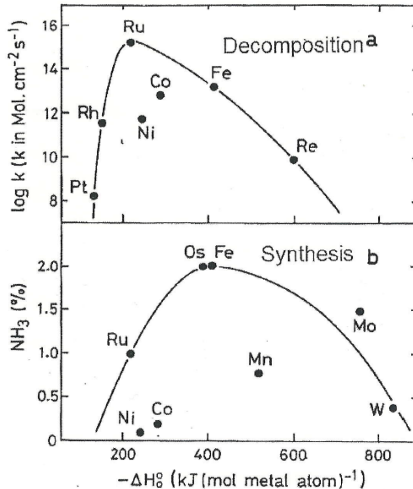
アンモニア分解(a)、合成(b)活性とM-O結合エネルギーの関係
