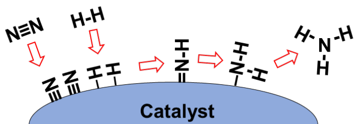
アンモニア生成反応機構
