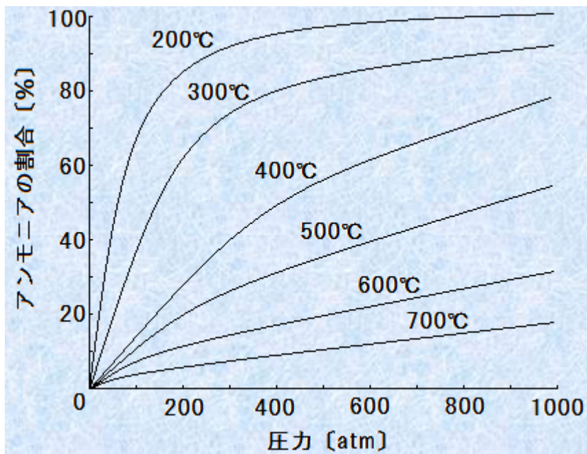
アンモニア生成平衡曲線
