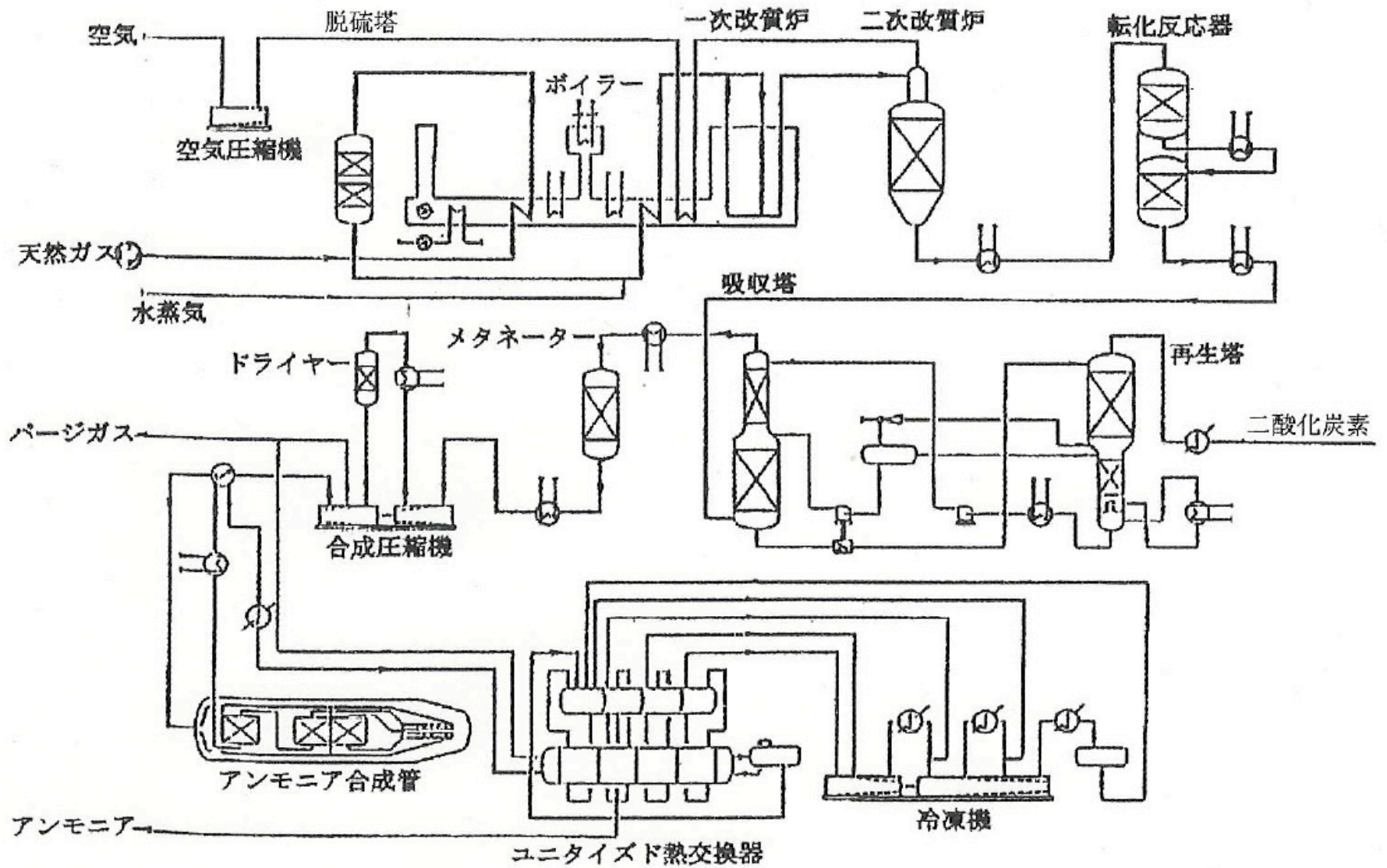
アンモニア合成プロセスフローシート (KBR法)
